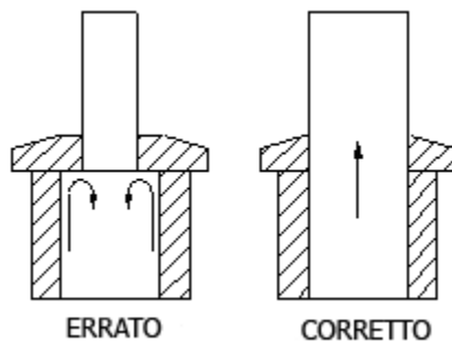
SEZIONE TUBO INSUFFICIENTE
